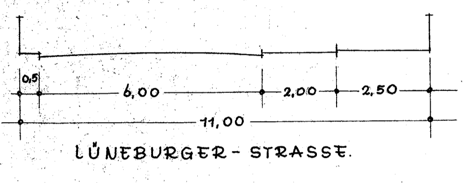
STRASSENSCHNITTE. M. 1:100
